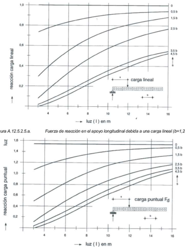
Figura A.12.5.2.5.b. Fuerza de reacción en el apoyo longitudinal debida a una carga puntual en el centro de vano ( b=1,20 m)
